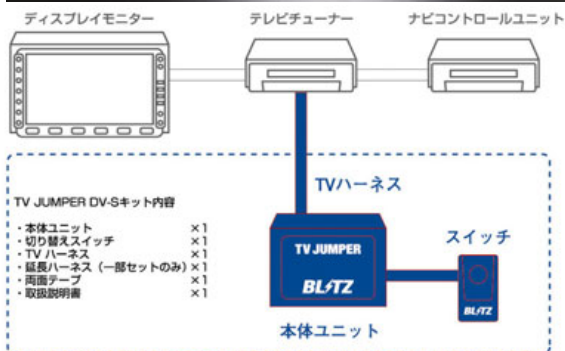
TV JUMPER DV-S システム構成図
