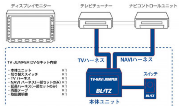
TV-NAVI JUMPER DV-S システム構成図
