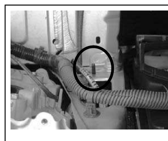
図6 ヒートプレート 取り付け用スタッド ボルト位置
