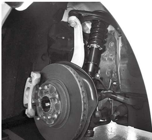
フロント右側(運転席側)取り付け状態
