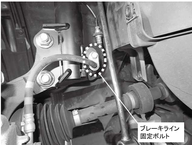
ブレーキライン固定ボルト 1カ所締め付け 締め付けトルク: 22N・m(2.2kgf・m)
