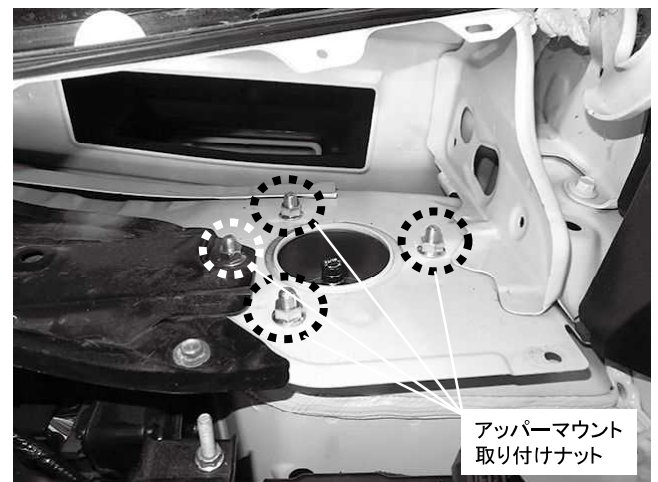
アッパーマウント取り付けナット 4カ所締め付け 締め付けトルク: 44N・m(4.5kgf・m) ※上写真はワイパーカウルを取り外している状態で ※製品付属のM10ナットを使用してください
