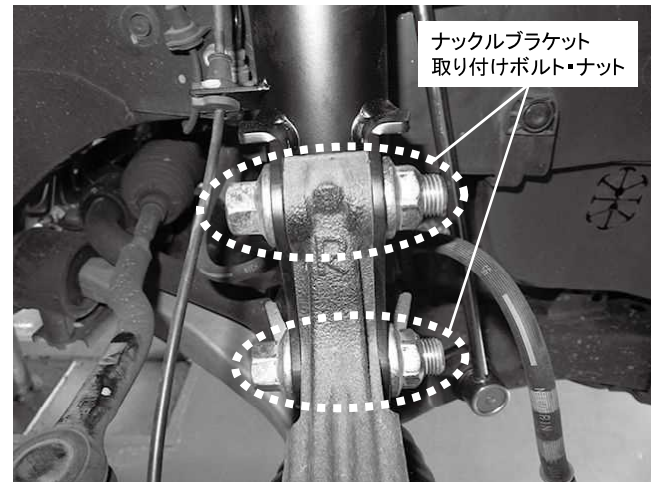
ナックルブラケット取り付けボルト・ナット 2カ所締め付け 締め付けトルク: 152N・m(15.5kgf・m) ※取り付け上部は長穴になっておりキャンバー調整が可能です
