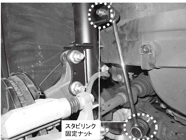
スタビリンク固定ナット 2カ所締め付け 締め付けトルク: 79N・m(8.0kgf・m) ※商品同梱スタビリンクを使用してください
