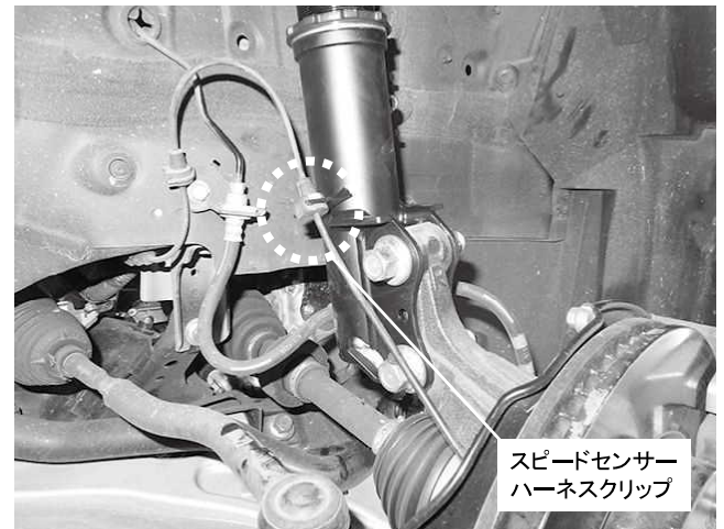
スピードセンサーハーネスクリップ 1カ所取り付け
