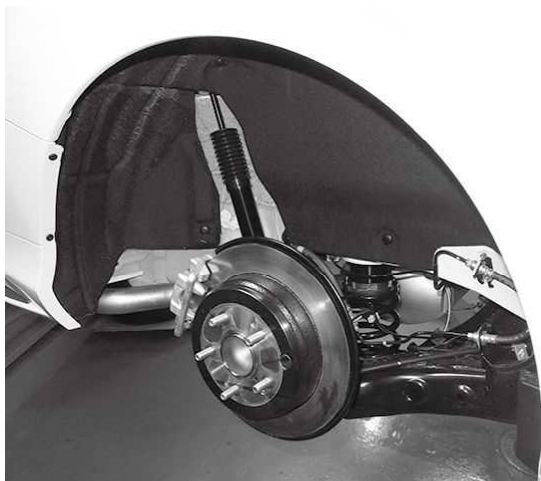
リア右側(運転席側)取り付け状態
