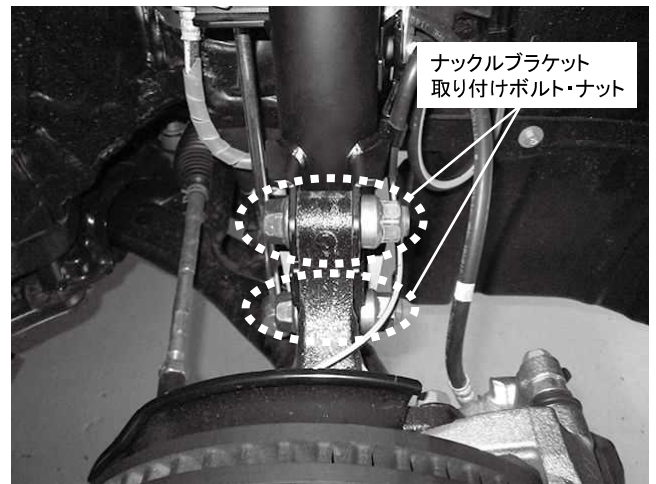
ナックルブラケット取り付けボルト・ナット 2カ所締め付け 締め付けトルク: 220N・m(22.4kgf・m)
