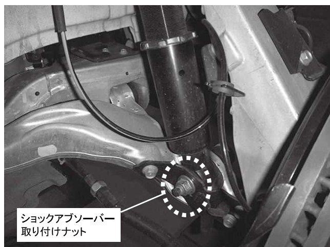
ショックアブソーバー下側取り付けナット 1カ所締め付け 締め付けトルク: 163N・m(17.0kgf・m)
