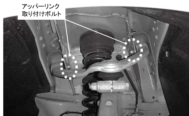
アッパーリンク取り付けボルト 2カ所締め付け 締め付けトルク: 54N・m(5.5kgf・m)
