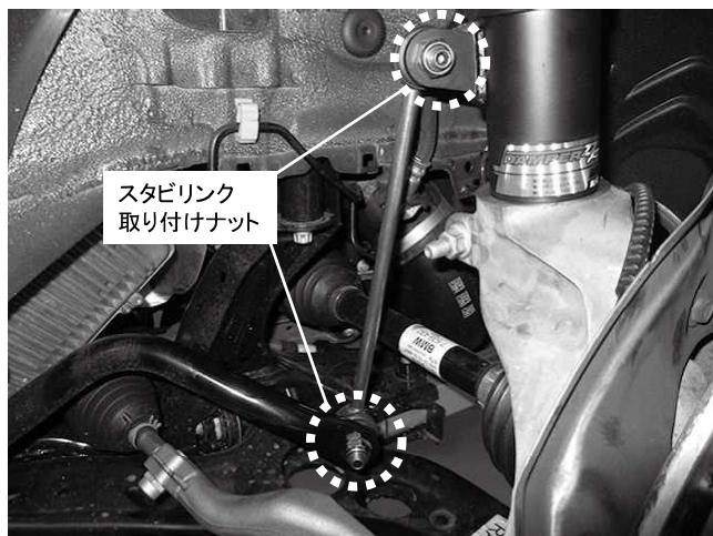
スタビリンク(キット付属品)取り付け ナット 2カ所締め付け 締め付けトルク: 60\text{N}\cdot\text{m} ( 6.0\text{kgf}\cdot\text{m} )
