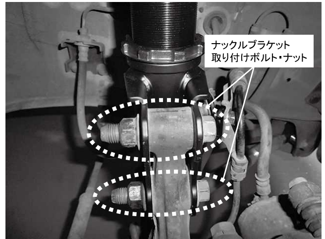
ナックルブラケット取り付けボルト・ナット 2カ所締め付け 締め付けトルク: 152N・m(15.5kgf・m)
