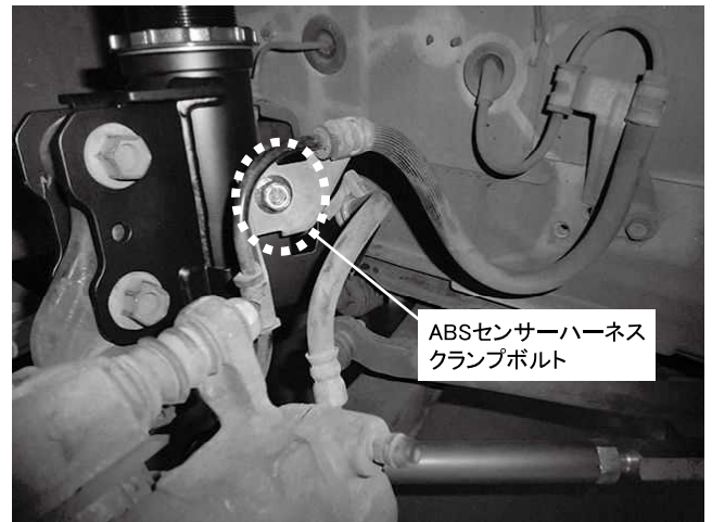
ABSセンサーハーネスクランプボルト 1カ所締め付け 締め付けトルク: 26N・m(2.7kgf・m)
