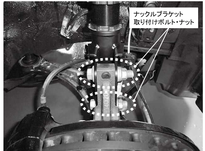
ナックルブラケット取り付けボルト・ナット 2カ所締め付け 締め付けトルク: 155N・m(15.8kgf・m)
