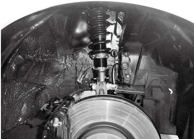
フロント右側(運転席側)取り付け状態
