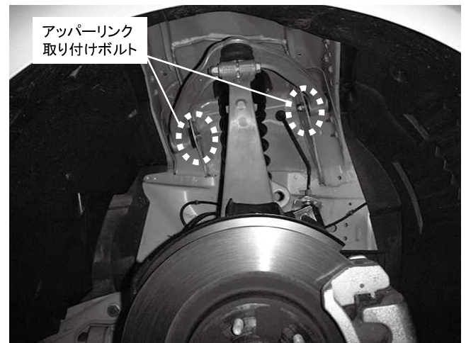
アッパーリンク 取り付けボルト 2カ所締め付け 締め付けトルク: 54N・m(5.5kgf・m)
