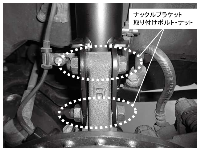
ナックルブラケット取り付けボルト・ナット 2カ所締め付け 締め付けトルク: 110N・m(11.0kgf・m)
