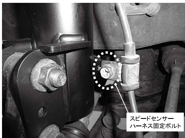
スピードセンサーハーネス固定ボルト 1カ所締め付け 締め付けトルク: 9.8N・m(1.0kgf・m) ※ネジ部に塗装がついて締め付けが渋い場合があります
