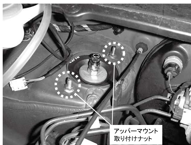
アッパーマウント取り付けナット 2カ所締め付け 締め付けトルク: 28N・m(2.9kgf・m) ※製品付属のM8ナットを使用してください
