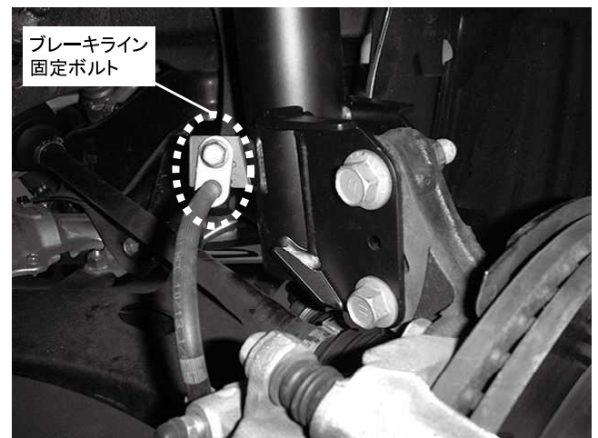
ブレーキライン固定ボルト 1カ所締め付け 締め付けトルク: 33N・m(3.4kgf・m) ※ネジ部に塗装がついて締め付けが渋い場合があります
