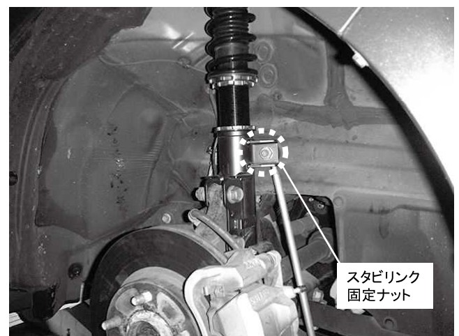
スタビリンク 固定ナット スタビリンク固定ナット 1カ所締め付け 締め付けトルク: 74N・m(7.5kgf・m)
