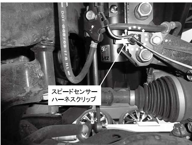
スピードセンサー ハーネスクリップ スピードセンサーハーネスクリップ取り付け ※クリップがブラケットに固定できない、またはハーネスが 突っ張ってしまう場合にはクリップをハーネスから取り外し、 クリップをロアブラケットに付けてからハーネスを取り付けてください
