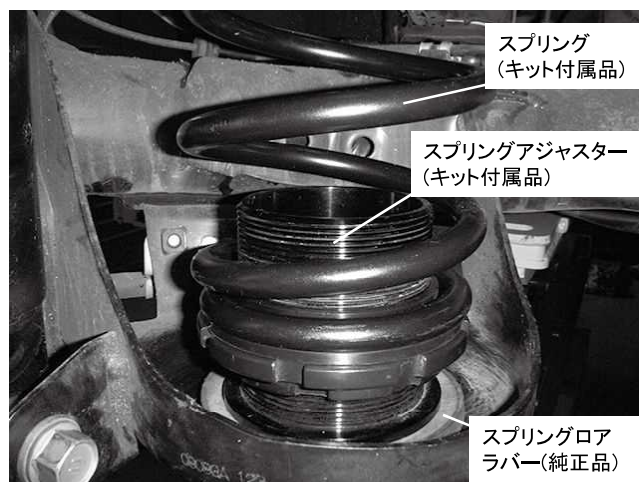
リアスプリング取り付け状態 ※スプリングアジャスター下部に純正スプリングロアラバー(インシュレーター)を取り付けてください
