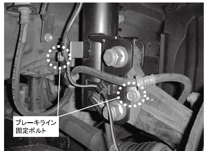
ブレーキライン 固定ボルト ブレーキライン固定ボルト 2カ所締め付け 締め付けトルク: 18.5N・m(1.9kgf・m) ※ネジ部に塗装がついて締め付けが渋い場合があります
