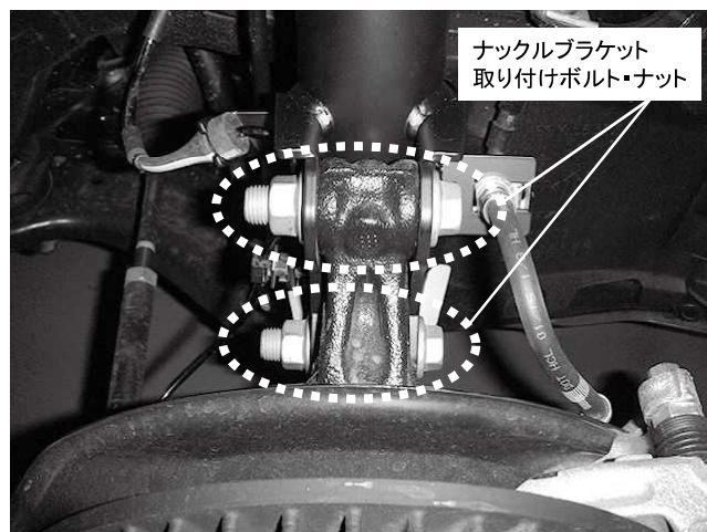
ナックルブラケット取り付けボルト・ナット 2カ所締め付け 締め付けトルク: 159N・m(16.2kgf・m) ※取り付け上部は長穴になっておりキャンバー調整が可能です
