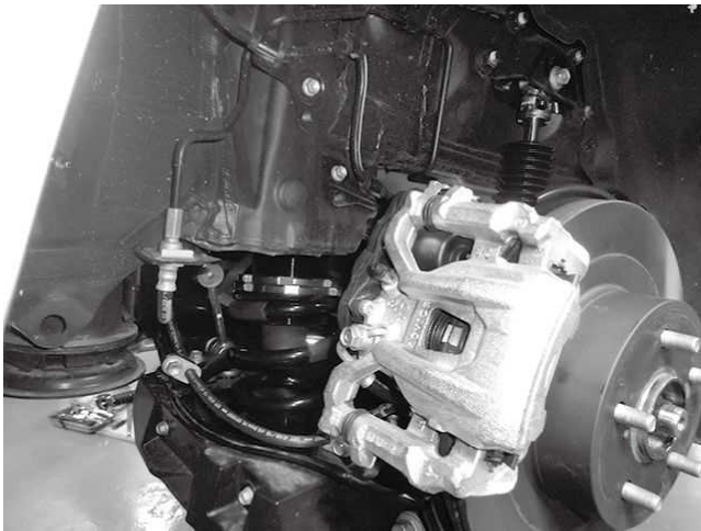
リア右側(運転席側)取り付け状態 ※ショック取り付け方向については 下写真を参照してください
