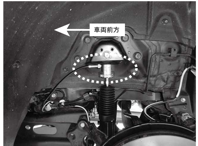
リアショックアブソーバー取り付け状態 ※モーター固定用フレキシブルアダプター ワイヤーは車両前方に向けて取り付けてください
