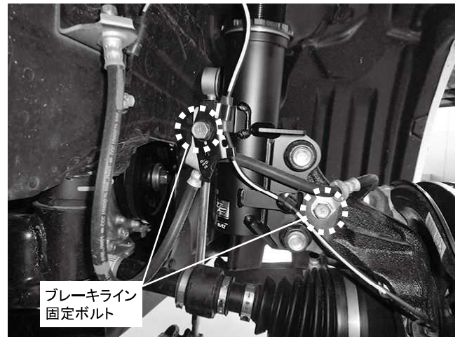
ブレーキライン固定ボルト 2カ所締め付け 締め付けトルク: 18.5N・m(1.9kgf・m) ※ネジ部に塗装がついて締め付けが渋い場合があります
