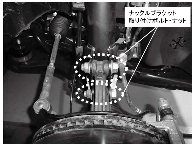
ナックルブラケット取り付けボルト・ナット 2カ所締め付け 締め付けトルク: 103N・m(10.5kgf・m) ※取り付け上部は長穴になっておりキャンバー調整が可能です
