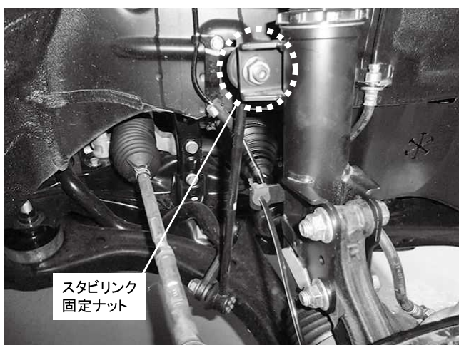
スタビリンク固定ナット 1カ所締め付け 締め付けトルク: 79N・m(8.1kgf・m)
