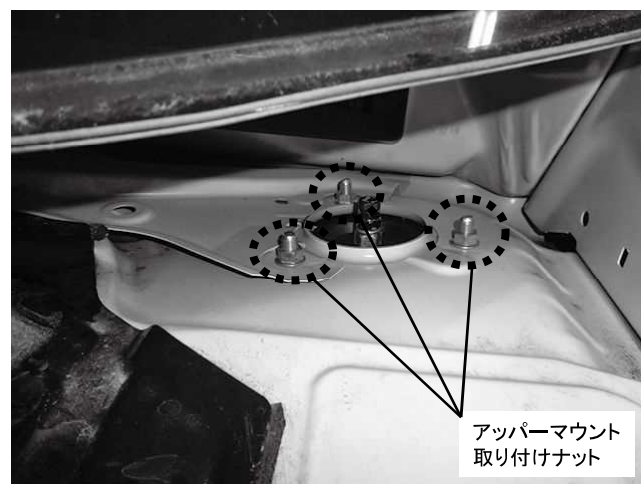
アッパーマウント取り付けナット 3カ所締め付け 締め付けトルク: 64N・m(6.5kgf・m) ※製品付属のM10ナットを使用してください
