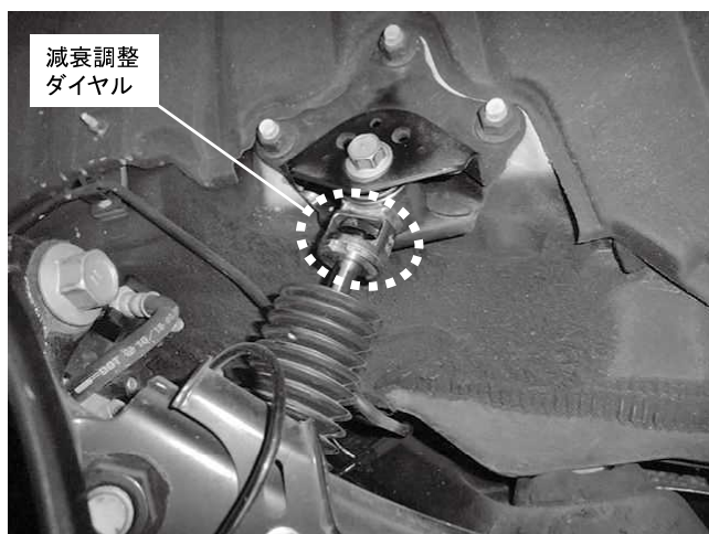
リアショックアブソーバー取り付け状態 ※減衰調整ダイヤルは構造上 リアショック上部についています
