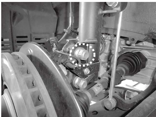
ショックアブソーバーナックルブラケット上側取り付け穴は 長穴になっており、キャンバー調整が可能です 左右で位置を合わせて取り付けてください
