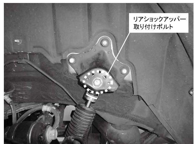
リアショックアッパース取り付けボルト 1カ所締め付け 締め付けトルク: 90N・m(9.2kgf・m)
