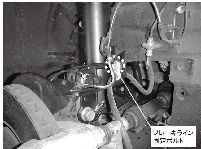
ブレーキライン固定ボルト 1カ所締め付け 締め付けトルク: 18.8N・m(1.9kgf・m) ※ネジ部に塗装がついて締め付けが渋い場合があります
