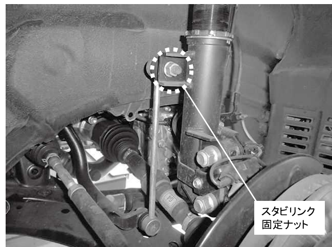
スタビリンク固定ナット 1カ所締め付け 締め付けトルク: 76N・m(7.8kgf・m)
