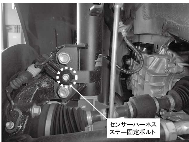
ブレーキライン固定ボルト 1カ所締め付け 締め付けトルク: 10.0N・m(1.0kgf・m) ※ネジ部に塗装がついて締め付けが渋い場合があります
