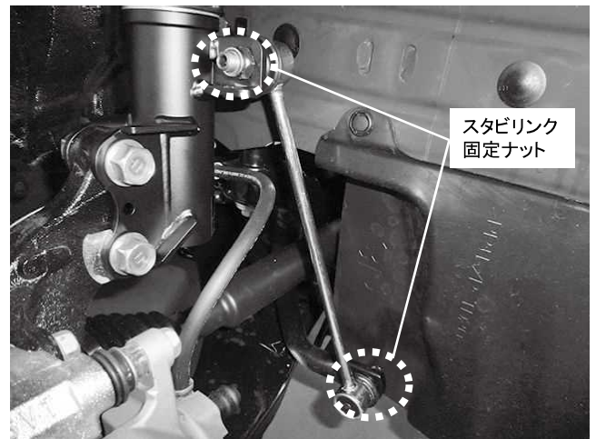
スタビリンク固定ナット 2カ所締め付け 締め付けトルク: 74N・m(7.5kgf・m) ※商品同梱スタビリンクを使用してください
