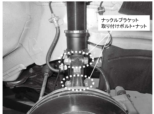
ナックルブラケット取り付けボルト・ナット 2カ所締め付け 締め付けトルク: 122N・m(12.4kgf・m)
