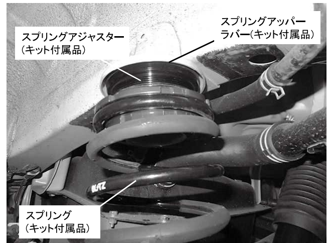
リアスプリングアッパー側取り付け状態 ※スプリングを取り付けの際、アジャスター上部に キット付属スプリングアッパーラバーを取り付けてください
