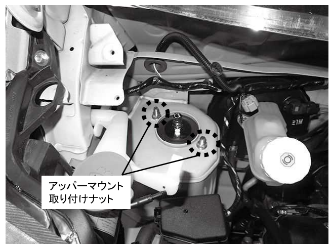
アッパーマウント取り付けナット 2カ所締め付け 締め付けトルク: 58N・m(5.9kgf・m) ※製品付属のM10ナットを使用してください
