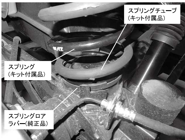
リアスプリングロア側取り付け状態 ※スプリングをリアアクスルに取り付けの際、 純正スプリングロアラバーを取り付けてください ※スプリングが線間密着する際、必要に応じてスプリング チューブを使用してください
