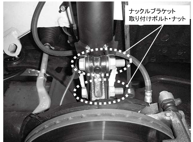
ナックルブラケット取り付けボルト・ナット 2カ所締め付け 締め付けトルク: 95.7N・m(9.7kgf・m)
