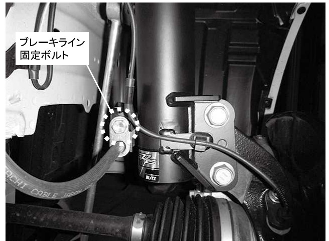
ブレーキライン固定ボルト 1カ所締め付け 締め付けトルク: 20.5N・m(2.1kgf・m) ※純正同様スピードセンサーハーネス固定ステーと 一緒に取り付けてください
