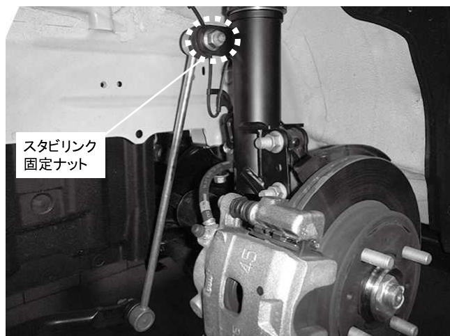
スタビリンク固定ナット 1ヵ所締め付け 締め付けトルク: 40\text{N}\cdot\text{m} ( 4.1\text{kgf}\cdot\text{m} )
