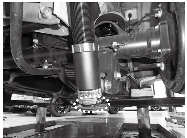
ショックアブソーバー全長を短くしていくと ロアブラケット下部よりシリンダーネジ部が出てきます 短くしすぎないように注意してください
