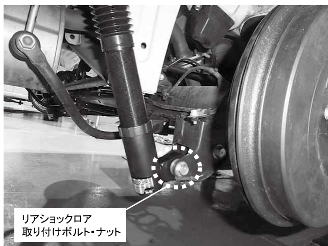
リアショックロア取り付けボルト・ナット 1カ所締め付け 締め付けトルク: 106N・m(10.8kgf・m)
