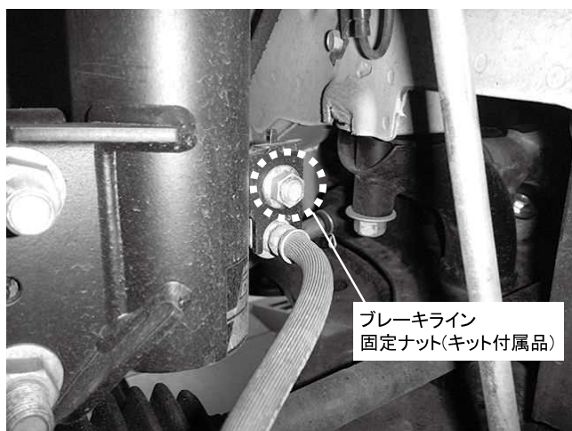
ブレーキライン取り付け状態 ブレーキラインの固定には純正のボルトとキット付属の ナットを使用して固定してください
