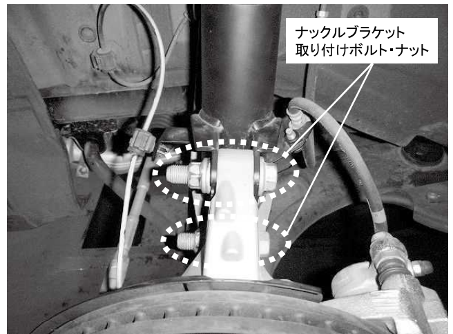
ナックルブラケット取り付けボルト・ナット 2カ所締め付け 締め付けトルク: 155\text{N}\cdot\text{m} ( 15.8\text{kgf}\cdot\text{m} )
