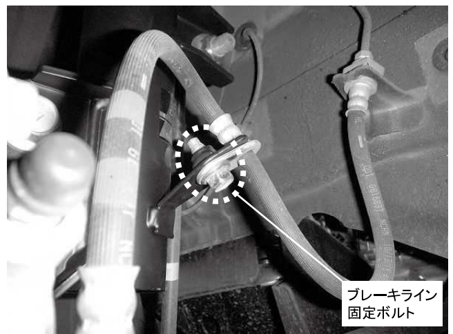
ブレーキライン固定ボルト 1カ所締め付け 締め付けトルク: 33\text{N}\cdot\text{m} ( 3.4\text{kgf}\cdot\text{m} ) ※ネジ部に塗装がついて締め付けが渋い場合があります
