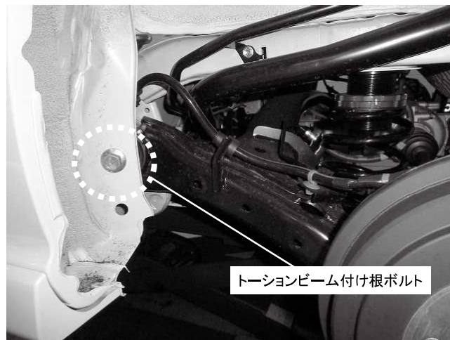
トーションビーム付け根ボルト 1カ所締め付け 締め付けトルク: 79N・m (8.0kgf・m)
