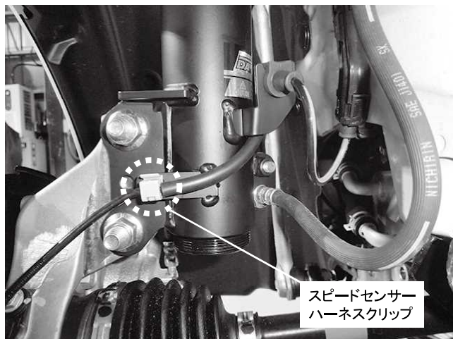
スピードセンサーのクリップ固定 クリップは純正品を取り外して使用してください
