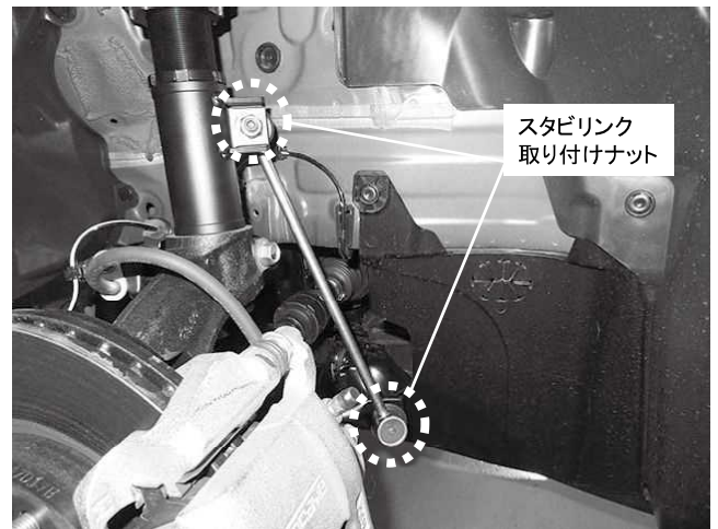
スタビリンク固定ナット 2ヵ所締め付け 締め付けトルク: 64\text{N}\cdot\text{m} ( 6.5\text{kgf}\cdot\text{m} ) ※商品同梱スタビリンクを使用してください
