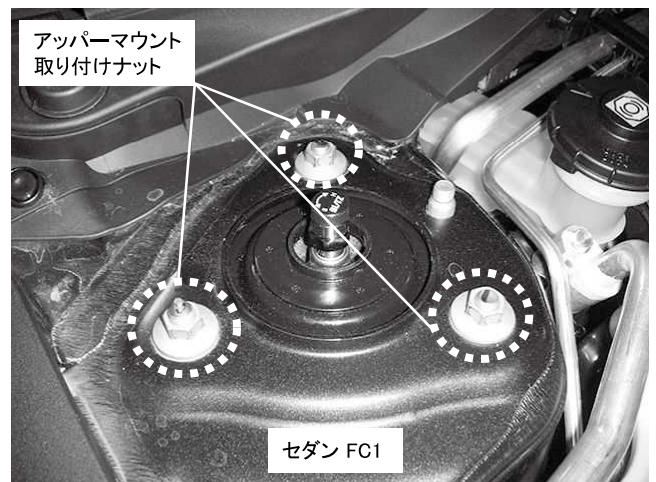
アッパーマウント取り付けナット 3ヵ所締め付け 締め付けトルク: 75\text{N}\cdot\text{m} ( 7.6\text{kgf}\cdot\text{m} ) ※ナットは純正品を使用してください
