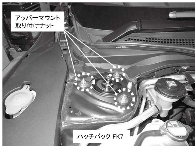
アッパーマウント取り付けナット 3ヵ所締め付け 締め付けトルク: 63\text{N}\cdot\text{m} ( 6.4\text{kgf}\cdot\text{m} ) ※ナットは純正品を使用してください
