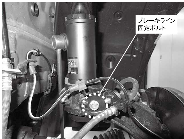
ブレーキライン固定ボルト 1ヵ所締め付け 締め付けトルク: 22\text{N}\cdot\text{m} ( 2.2\text{kgf}\cdot\text{m} )
