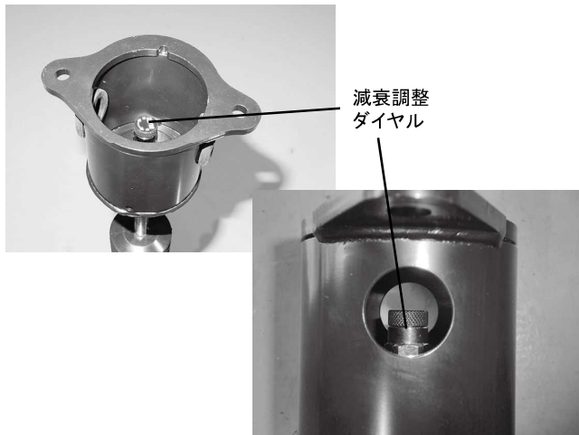
減衰力調整ダイヤルはアッパーマウント内部に配置されます 車両にショックを取り付け前の調整をお勧めします
