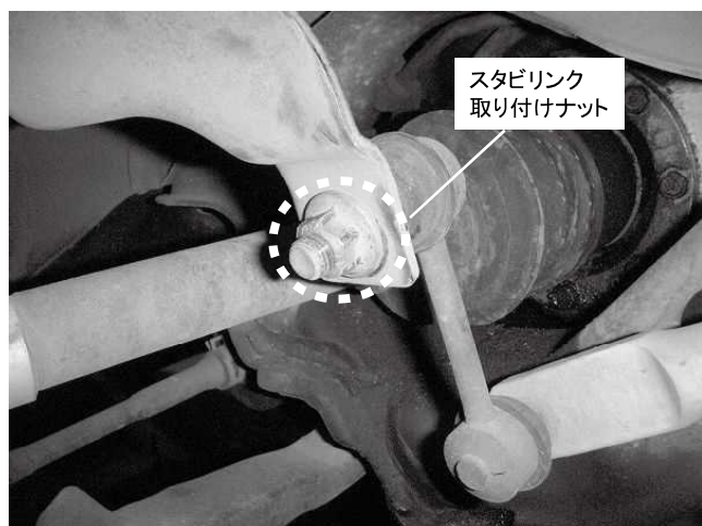
スタビリンク取り付けナット 1ヵ所締め付け 締め付けトルク: 47\text{N}\cdot\text{m} ( 4.8\text{kgf}\cdot\text{m} )
