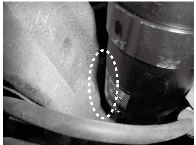
ナット締め付け後、ロアブラケットとナックルの 干渉がないか確認してください。
