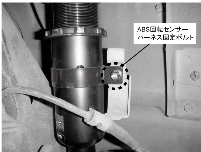
ABS回転センサーハーネス固定ボルト 1カ所締め付け 締め付けトルク: 6.0N・m(0.6kgf・m)
