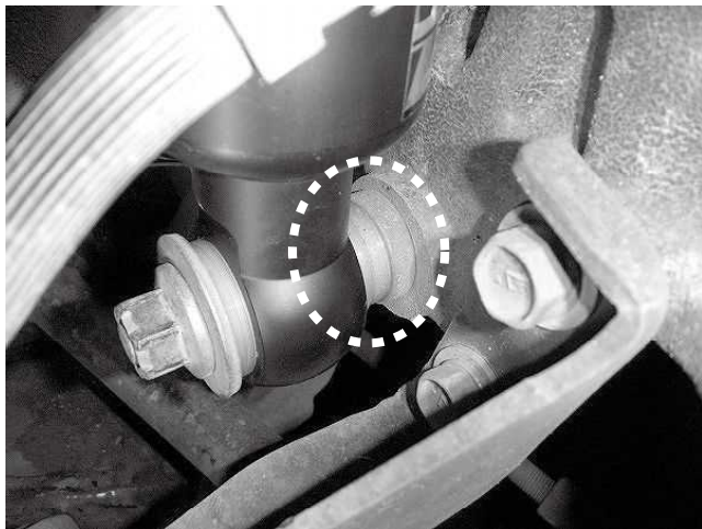
フロントロアブラケット取り付けの際、 ブッシュの長いほうをナックル側にして 取り付けてください。
