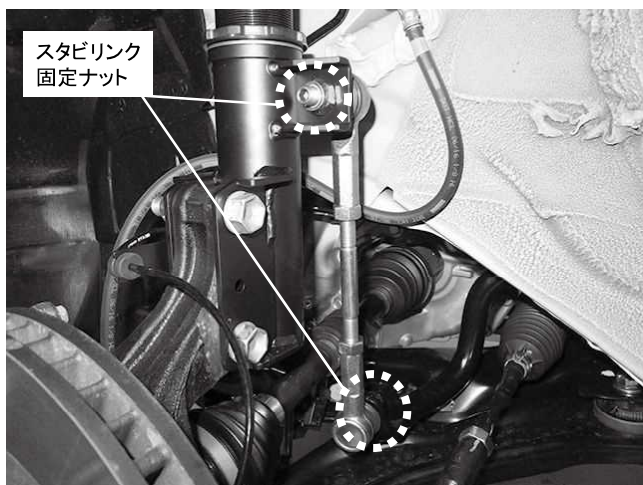
スタビリンク固定ナット 2カ所締め付け 締め付けトルク: 84\text{N}\cdot\text{m} ( 8.6\text{kgf}\cdot\text{m} ) ※調整式スタビリンクになっているので長さを合わせて ナットを締め付け固定してください 締め付けトルク: 60\text{N}\cdot\text{m} ( 6.1\text{kgf}\cdot\text{m} )
