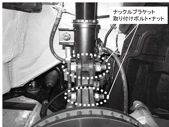
ナックルブラケット取り付けボルト・ナット 2カ所締め付け
