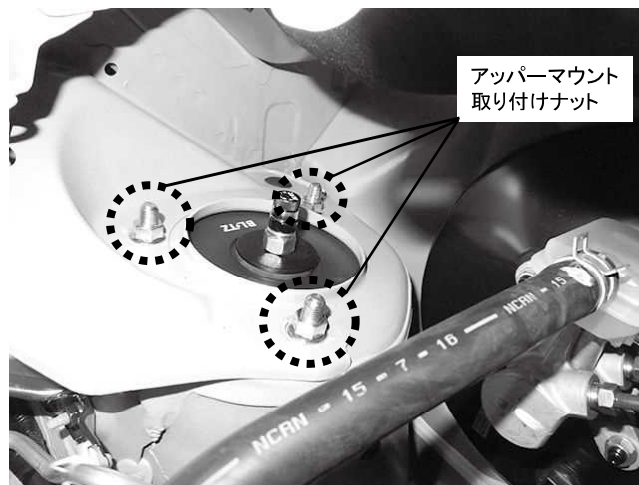
アッパーマウント取り付けナット 3カ所締め付け 締め付けトルク: 19\text{N}\cdot\text{m} ( 1.9\text{kgf}\cdot\text{m} ) ※製品付属のM10ナットを使用してください
