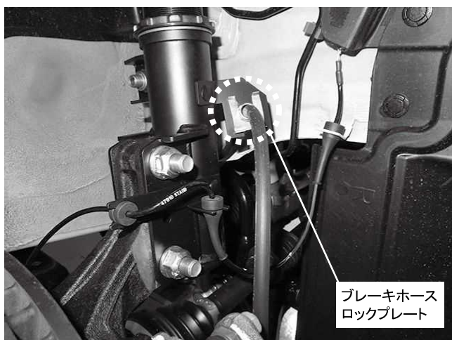
ブレーキホースロックプレート取り付け ※ブレーキホースと他部品が干渉していないか 確認してください
