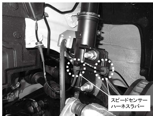
スピードセンサーハーネススライダー 2カ所取り付け ※スピードセンサーハーネスが突っ張っていたり しないか確認してください
