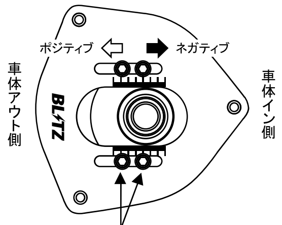
調整用ネジ
