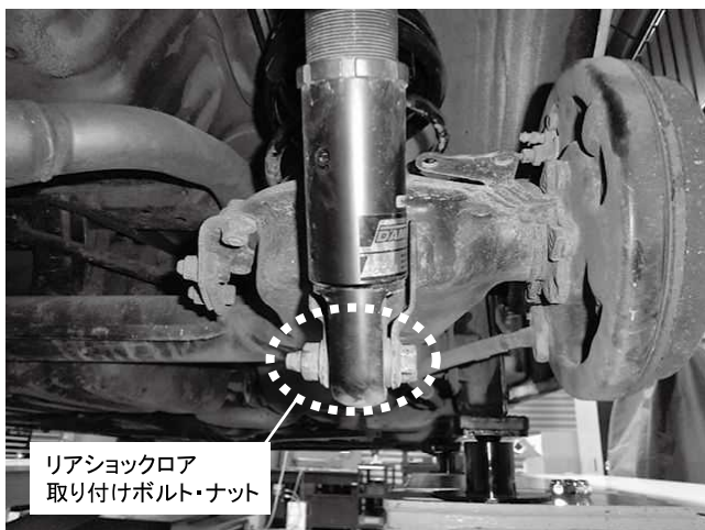
リアショックロー取り付けボルト・ナット 1カ所締め付け 締め付けトルク: 93N・m(9.5kgf・m)
