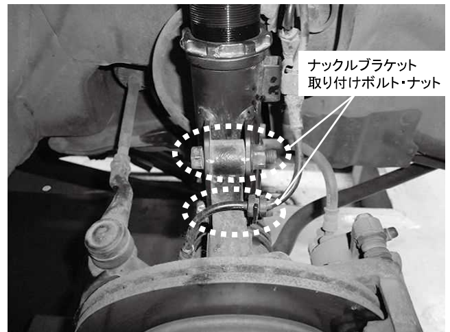
ナックルブラケット取り付けボルト・ナット 2カ所締め付け 締め付けトルク: 108N・m(10.8kgf・m)
