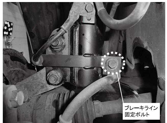
ブレーキライン固定ボルト・ナット 1カ所締め付け 締め付けトルク: 29N・m(3.0kgf・m)
