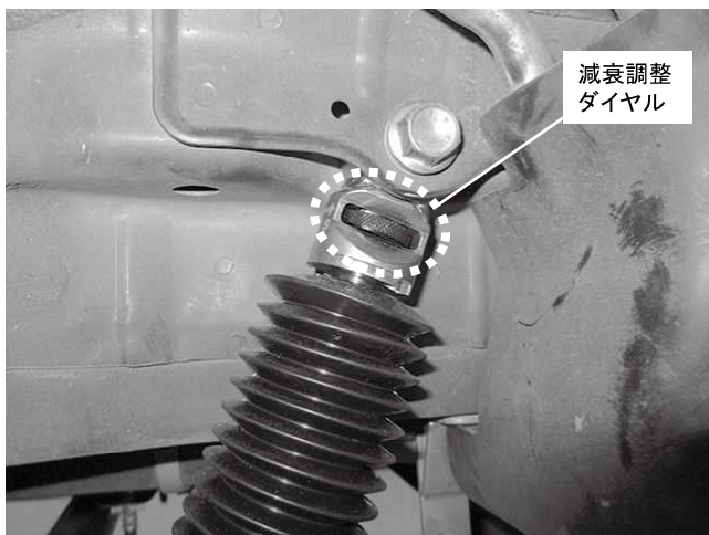
減衰調整ダイヤルはタイヤハウス内 ショックアブソーバー上部に配置されます
