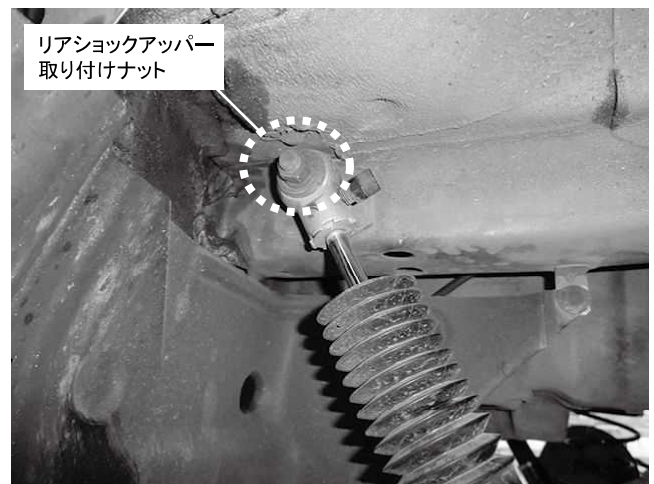
リアショックアッパ取り付けナット 1カ所締め付け 締め付けトルク: 78.5N・m(8.0kgf・m) ※純正ワッシャーも使用して取り付けください ※減衰調整ダイヤルの形状は製品と異なります
