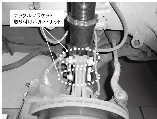
ナックルブラケット取り付けボルト・ナット 2カ所締め付け 締め付けトルク: 96N・m(9.79kgf・m)
