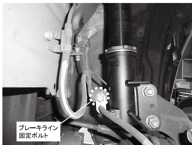
ブレーキライン固定ボルト・ナット 1カ所締め付け 締め付けトルク: 21N・m(2.14kgf・m) ブレーキラインの固定には純正ボルトとキット付属の ナットを使用して固定してください
