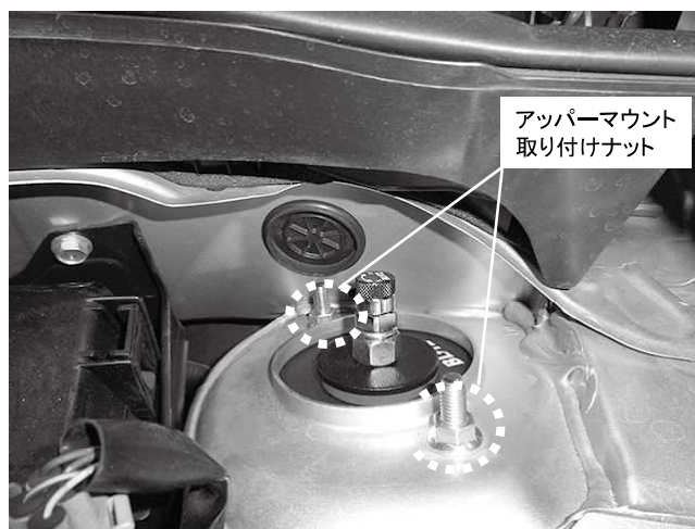
アップアマウント取り付けナット 2カ所締め付け 締め付けトルク: 27N・m(2.75kgf・m) ※製品付属のM8ナットを使用してください
