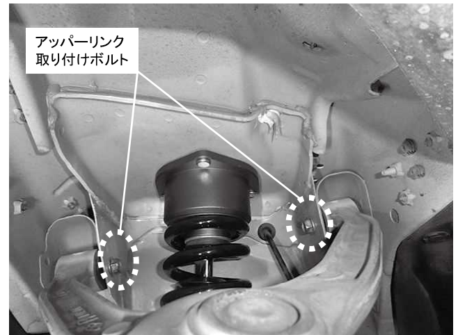
アッパーリンク取り付けボルト 2カ所締め付け 締め付けトルク: 54\text{N}\cdot\text{m} ( 5.5\text{kgf}\cdot\text{m} )
