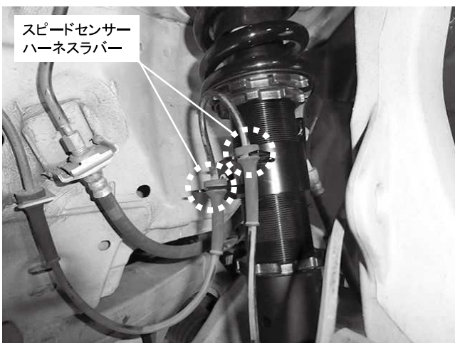
スピードセンサーハーネスラバー 2カ所取り付け ※スピードセンサーハーネスが突っ張っていたりしないか確認してください
