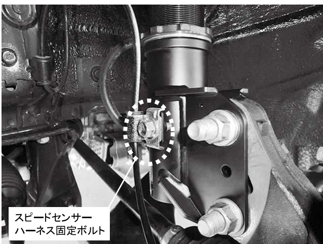
スピードセンサー ハーネス固定ボルト スピードセンサーハーネス固定ボルト 1カ所締め付け 締め付けトルク: 20N・m(2.0kgf・m) ※ネジ部に塗装がついて締め付けが渋い場合があります
