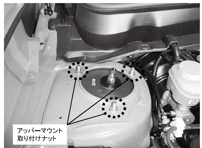
アップアマウント 取り付けナット アップアマウント取り付けナット 3カ所締め付け 締め付けトルク: 25N・m(2.5kgf・m) ※アップアマウント取り付け時シャフトのセンターが オフセットしているため、上写真を参照しシャフトが 車両内側にくるよう取り付けてください
