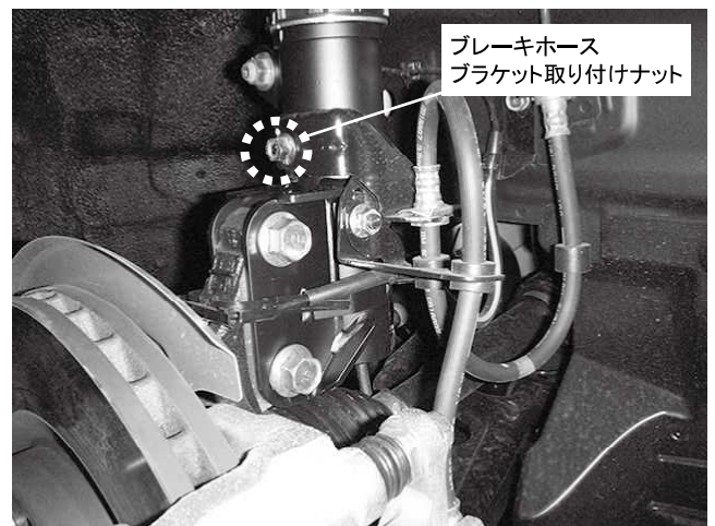
ブレーキホースブラケット取り付けナット 1カ所締め付け 締め付けトルク: 13N・m(1.3kgf・m)
