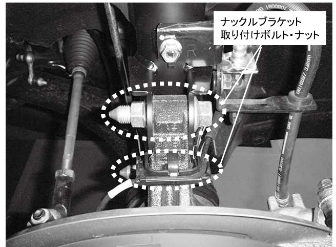
ナックルブラケット 取り付けボルト・ナット 2カ所締め付け 締め付けトルク: 120N・m(12.1kgf・m)
