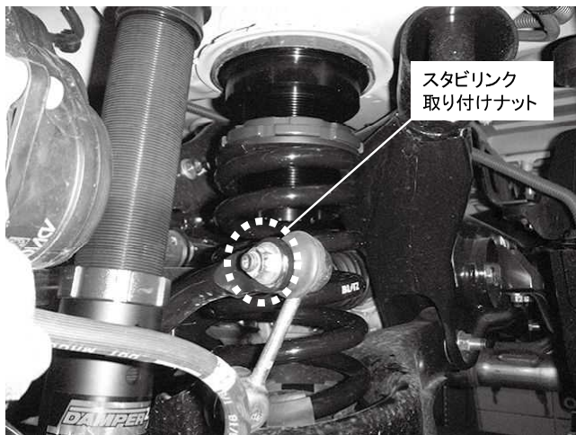
スタビリンク取り付けナット 1カ所締め付け 締め付けトルク: 39\text{N}\cdot\text{m} ( 3.9\text{kgf}\cdot\text{m} )
