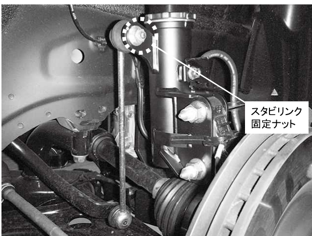
スタビリンク固定ナット 1カ所締め付け 締め付けトルク: 39N・m(3.9kgf・m)
