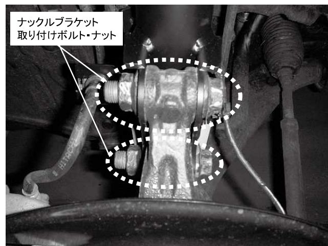
ナックルブラケット取り付けボルト・ナット 2カ所締め付け 締め付けトルク: 245N・m(25.0kgf・m) ※取り付け上部は長穴になっておりキャンバー調整が可能です
