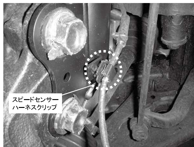
スピードセンサーハーネスクリップ 1カ所取り付け。この時、ハーネスが 突っ張らないように位置を調整してください。
