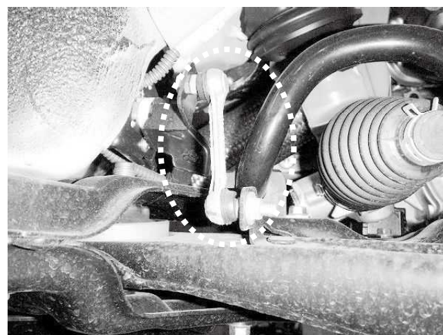
フロント右側(運転席側)のロアアームには、 ハイトセンサーが取り付けられています 作業時注意してください
