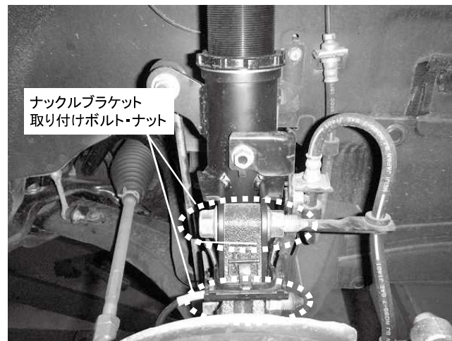
ナックルブラケット取り付けボルト・ナット 2カ所締め付け 締め付けトルク: 110N・m(11.2kgf・m)
