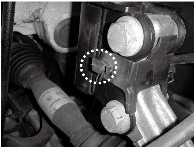
ブレーキホースブラケット取り付け 左右1カ所 ※しっかり奥まで差し込んで、 抜けないことを確認してください
