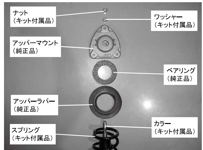
上写真を参照し、純正部品を キットに組みつけてください
