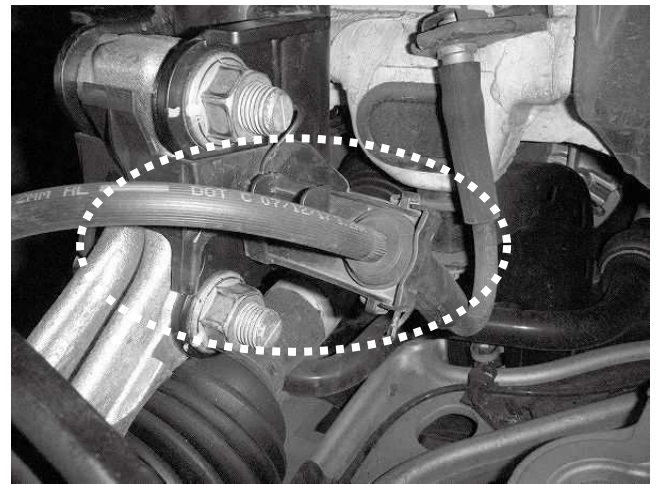
ブレーキホースブラケットを取り付けした際、 ブレーキホースが突っ張っている場合は、 ホースの固定位置を調整し突っ張りや、干渉がないか確認してください 無理に引っ張るとブラケットやホースが破損する 場合がありますので注意してください
