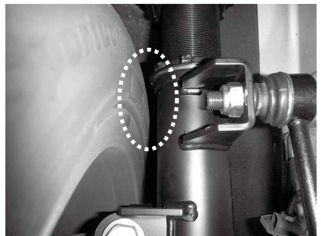
タイヤ取り付け後、ブラケットとタイヤ・ホイールが 干渉していないか確認をしてください ※写真は18インチ7.5J INSET52の 純正ホイール装着時のクリアランスになります
