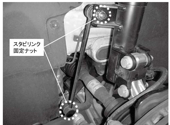
スタビリンク(キット付属品)取り付けナット 2カ所締め付け
