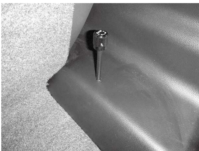
減衰延長ダイヤル取り付け状態(運転席側) ※内装パネルに穴あけ加工をして 取り付けています
