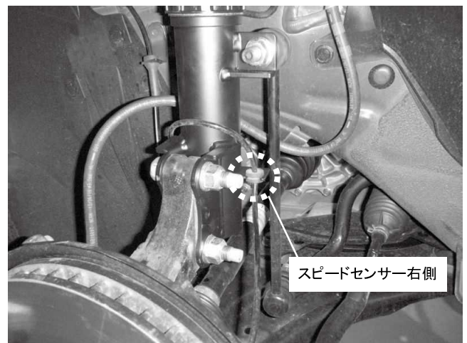
スピードセンサー右側 1カ所取り付け
