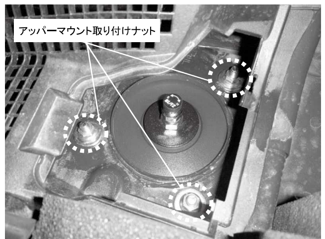
アッパーマウント取り付けナット 3カ所取り付け 締め付けトルク: 16\text{N}\cdot\text{m} ( 1.6\text{kgf}\cdot\text{m} ) ※キット付属のワッシャーを入れてから M8ナットを締め付けてください
