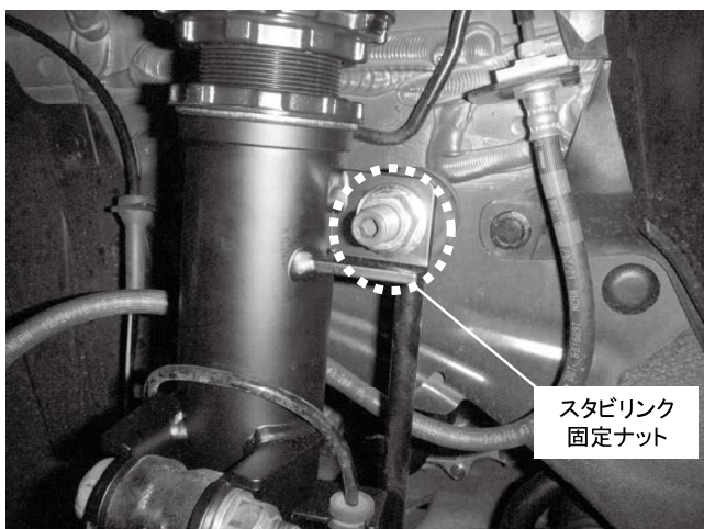
スタビリンク固定ナット 1カ所締め付け 締め付けトルク: 84\text{N}\cdot\text{m} ( 8.6\text{kgf}\cdot\text{m} )
