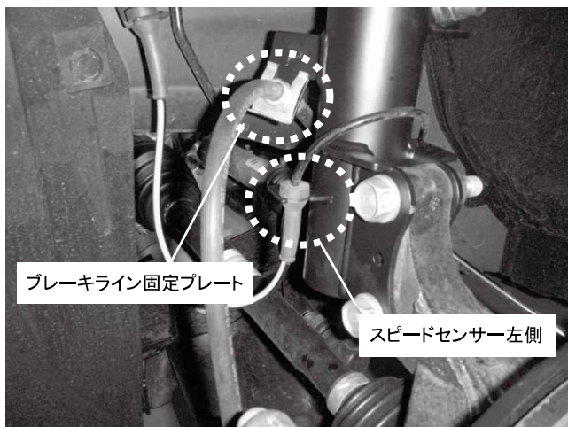
ブレーキライン固定プレート 1カ所取り付け スピードセンサー左側 1カ所取り付け
