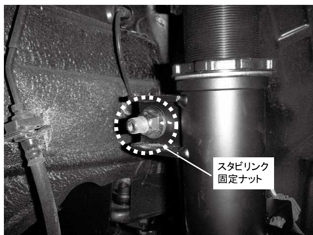
スタビリンク固定ナット 1カ所締め付け 締め付けトルク: 60N・m (6.1kgf・m)
