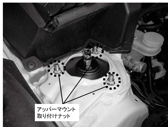
アッパーマウント取り付けナット 3カ所締め付け 締め付けトルク: 32N・m (3.3kgf・m) ※製品付属のM10ナットを使用してください
