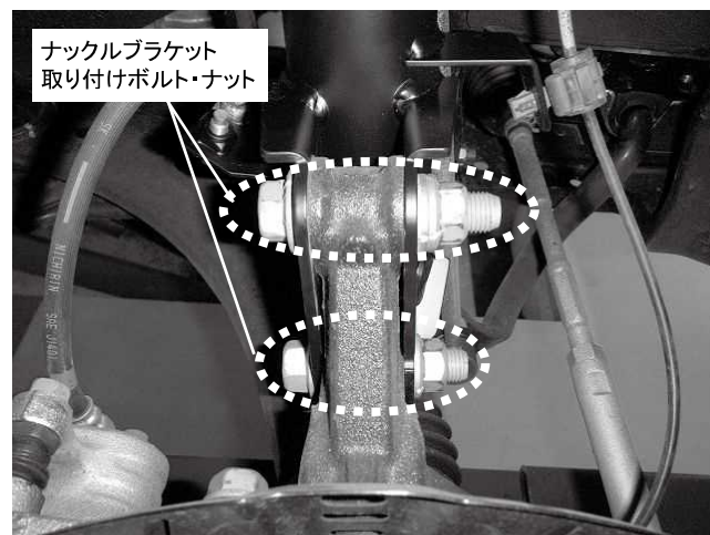
ナックルブラケット取り付けボルト・ナット 2カ所締め付け 締め付けトルク: 155N・m (15.8kgf・m) ※ワッシャーも純正同様に付けてください
