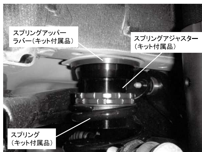
リアスプリング取り付け状態 (アッパー側) ※写真はAWD車の取り付け状態になります 2WDも同様取り付け方法です
