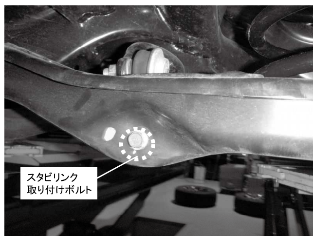
スタビリンク取り付けボルト(2WD) 1カ所締め付け 締め付けトルク: 40\text{N}\cdot\text{m} ( 4.1\text{kgf}\cdot\text{m} )
