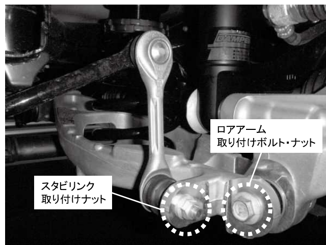
ロアアーム取り付けボルト・ナット(AWD車) 1カ所締め付け 締め付けトルク: 58\text{N}\cdot\text{m} ( 5.9\text{kgf}\cdot\text{m} ) スタビリンク取り付けナット(AWD車) 1カ所締め付け 締め付けトルク: 58\text{N}\cdot\text{m} ( 5.9\text{kgf}\cdot\text{m} )
