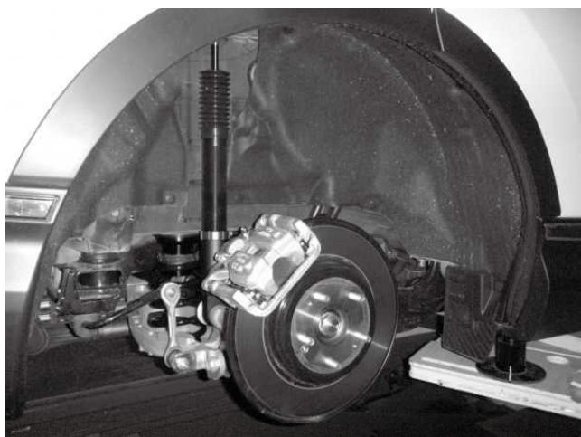
リア右側(運転席側)取り付け状態 ※写真はAWD車の取り付け状態になります
