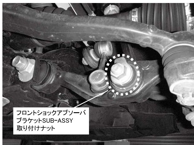
フロントショックアブソーバブラケットSUB-ASSY 取り付けナット 1カ所締め付け 締め付けトルク: 108N・m(11.0kgf・m)
