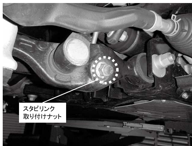
スタビリンク取り付けナット 1カ所締め付け 締め付けトルク: 125N・m(12.7kgf・m)
