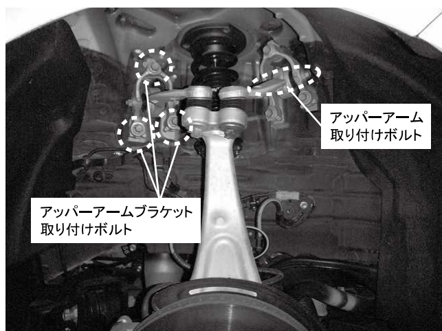
アッパーアームブラケット取り付けボルト 左右6カ所締め付け 締め付けトルク: 40N・m(4.1kgf・m) アッパーアーム取り付けボルト・ナット 左右2カ所締め付け 締め付けトルク: 45N・m(4.6kgf・m)
