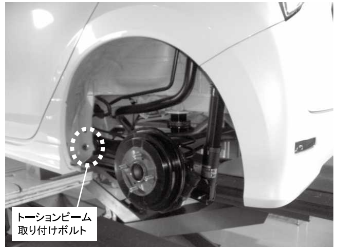
トーションビーム付け根ボルト
