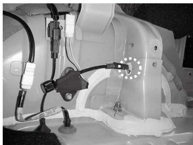
ボディの穴あけ加工例 加工せずに取り付けは可能ですが、 減衰調整の際はショックアブソーバーの 脱着が必要になります
