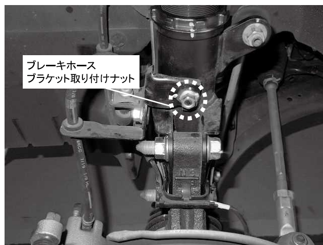
ブレーキホースブラケット取り付けナット 1カ所締め付け 締め付けトルク: 13\text{N}\cdot\text{m} ( 1.3\text{kgf}\cdot\text{m} )
