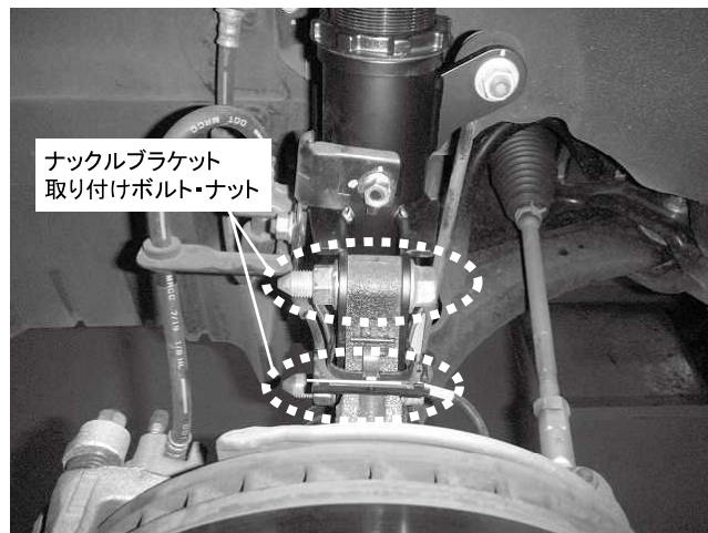
ナックルブラケット取り付けボルト・ナット 2カ所締め付け 締め付けトルク: 110\text{N}\cdot\text{m} ( 11.2\text{kgf}\cdot\text{m} )
