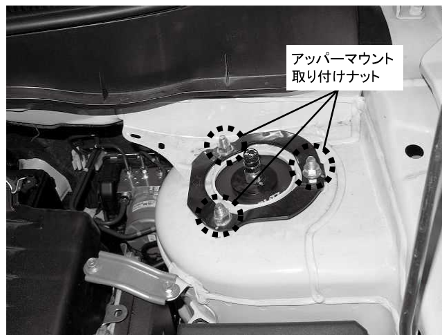
アッパーマウント取り付けナット 3カ所締め付け 締め付けトルク: 45\text{N}\cdot\text{m} ( 4.5\text{kgf}\cdot\text{m} ) ※製品付属のM10ナットを使用してください
