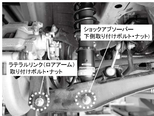
ショックアブソーバー 下側取り付けボルト・ナット ラテラルリンク(ロアアーム) 取り付けボルト・ナット ショックアブソーバー下側取り付けボルト・ナット 1カ所締め付け 締め付けトルク: 71N・m(7.2kgf・m) ラテラルリンク(ロアアーム)取り付けボルト・ナット 1カ所締め付け 締め付けトルク: 71N・m(7.2kgf・m)
