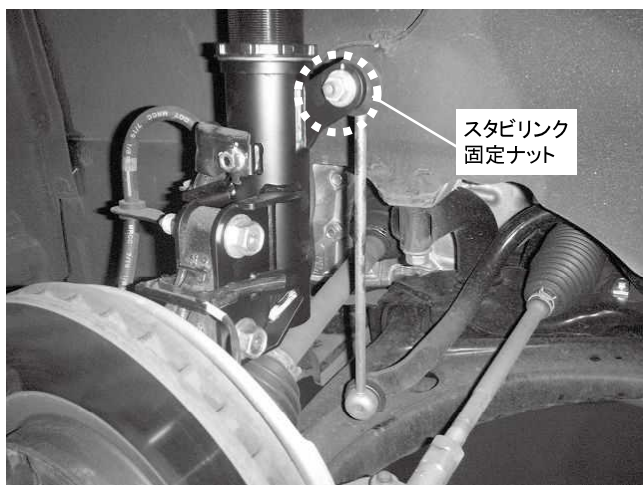
スタビリンク固定ナット 1カ所締め付け 締め付けトルク: 39\text{N}\cdot\text{m} ( 3.9\text{kgf}\cdot\text{m} )
