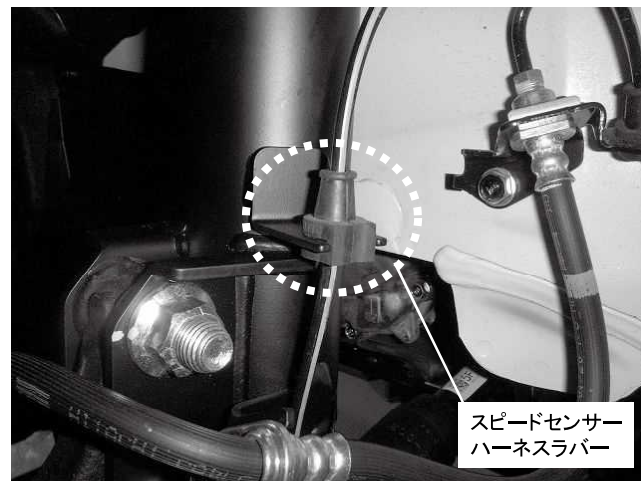
スピードセンサーのラバー固定 ※ハーネスがクリップに固定できない、またはハーネスが 突っ張ってしまう場合には潤滑油を使用しラバーの位置を ハーネスの上部にずらして固定してください
