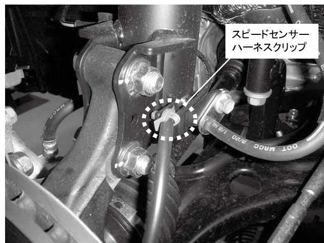
スピードセンサーハーネスクリップ固定 クリップは純正品を取り外して使用してください
