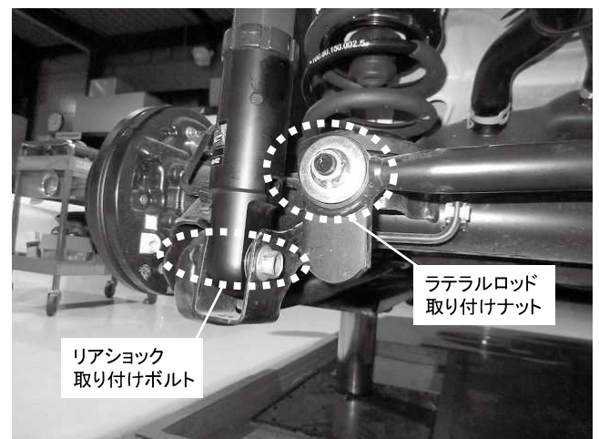
リアショック取り付けボルト
