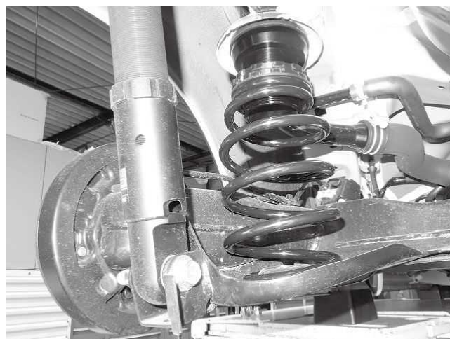
スプリング取り付け状態
