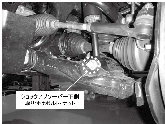
ショックアブソーバー下側取り付けボルト・ナット 1カ所締め付け 締め付けトルク: 95\text{N}\cdot\text{m} ( 9.7\text{kgf}\cdot\text{m} )
