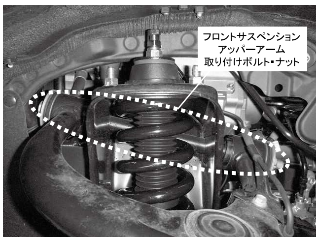
フロントサスペンションアッパーアーム 取り付けボルト・ナット 1カ所締め付け 締め付けトルク: 115\text{N}\cdot\text{m} ( 11.7\text{kgf}\cdot\text{m} )
