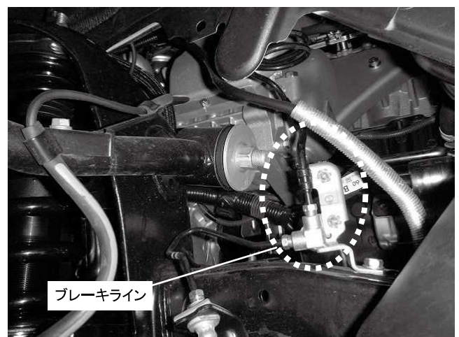
フロントサスペンションアッパーアームの ボルト・ナットを締め付ける際、 ブレーキラインの破損に注意してください
