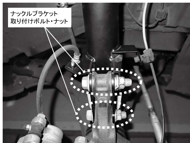
ナックルブラケット取り付けボルト・ナット 2カ所締め付け 締め付けトルク: 155N・m (15.8kgf・m) ※ワッシャーも純正同様に取付けてください
