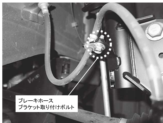
ブレーキホースブラケット取り付けボルト 1カ所締め付け 締め付けトルク: 33N・m (3.4kgf・m)
