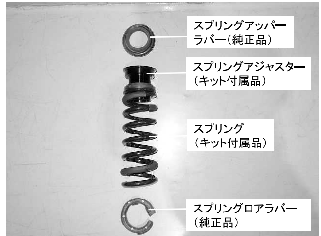
上写真を参照し、スプリングを車両に取り付けください
