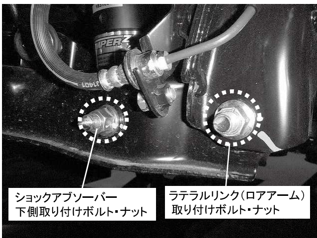
ショックアブソーバー下側取り付けボルト・ナット 1カ所締め付け 締め付けトルク: 71N・m (7.2kgf・m) ラテラルリンク(ロアアーム)取り付けボルト・ナット 1カ所締め付け 締め付けトルク: 71N・m (7.2kgf・m)
