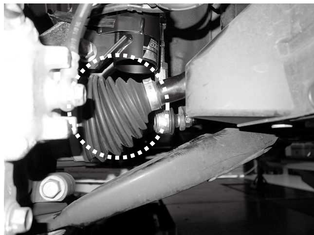
フロント右(運転席)アウト側のドライブシャフトとブーツの状態になります ※ドライブシャフトの傾き、ブラケットとの干渉がないか確認してください ※リフトアップすることでドライブシャフトブーツに通常よりも多く負担がかかりますので、破損していないか定期的に確認を行ってください ※写真は基準車高(寸法)の0G時状態です
