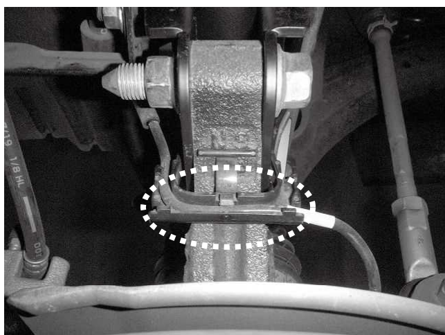
黒い樹脂は、そのまま利用します 取り外し際、割らないように注意してください
