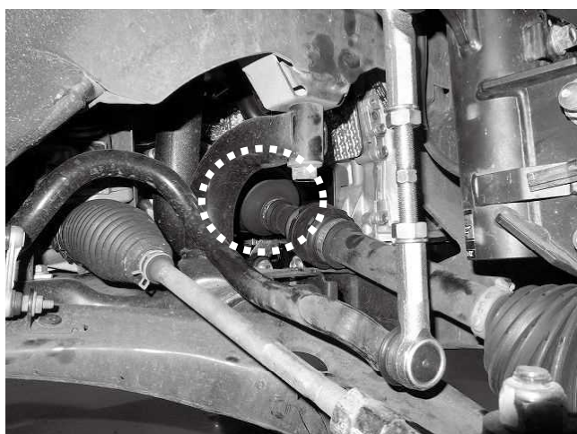
フロント右(運転席)イン側のドライブシャフトとブーツの状態になります ※ドライブシャフトの傾きを確認してください ※リフトアップすることでドライブシャフトブーツに通常よりも多く負担がかかりますので、破損していないか定期的に確認を行ってください ※写真は基準車高(寸法)の0G時状態です
