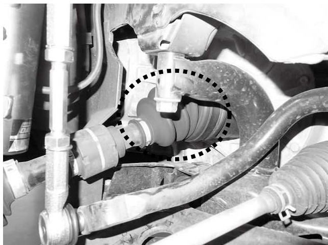
フロント左(助手席)イン側のドライブシャフトとブーツの状態になります ※ドライブシャフトの傾きを確認してください ※リフトアップすることでドライブシャフトブーツに通常よりも多く負担がかかりますので、破損していないか定期的に確認を行ってください ※写真は基準車高(寸法)の0G時状態です
