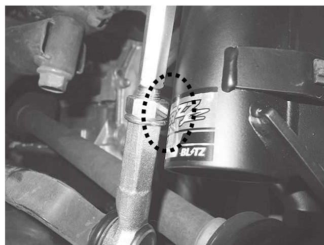
ステアリングを切るとスタビリンクとロアブラケット背面との クリアランスが狭くなります ※上写真はCV5W 0G時 その際は次ページ写真のようにスタビリンク上部に 製品同梱のワッシャーを入れてください
